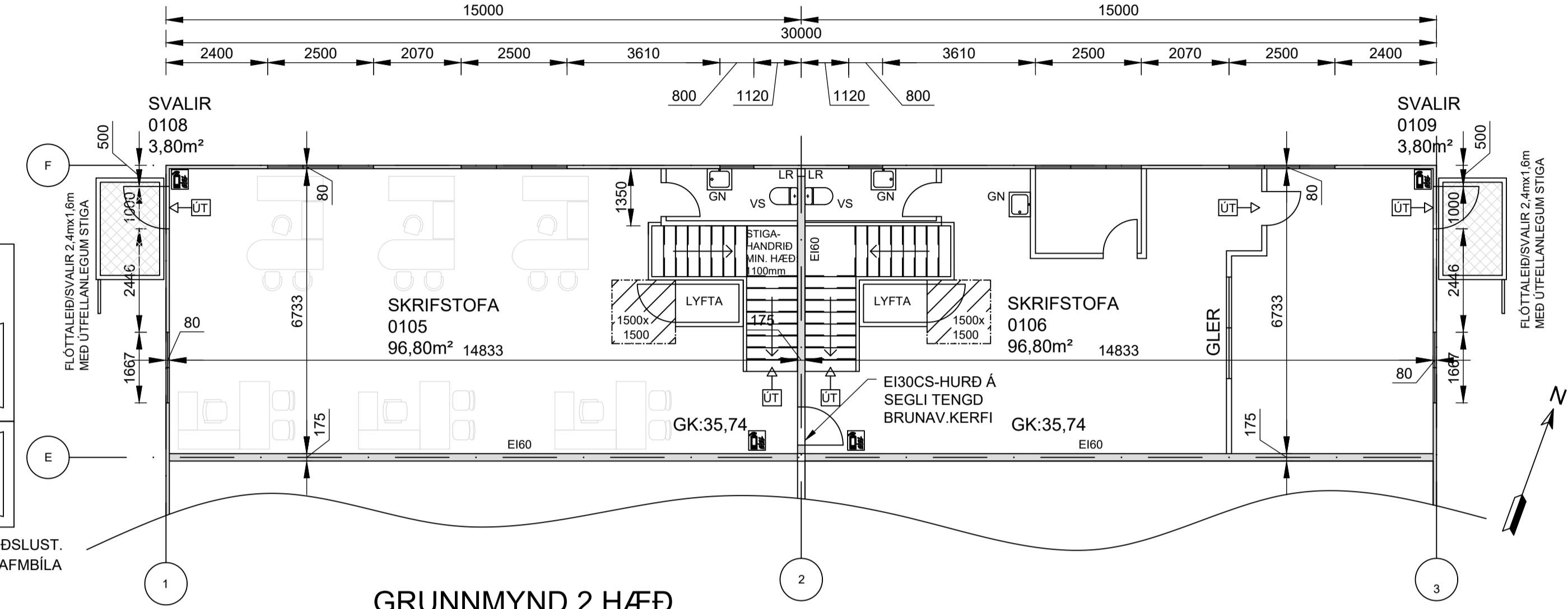
GRUNNMYND 2.HÆÐ 1:100 (A1)
